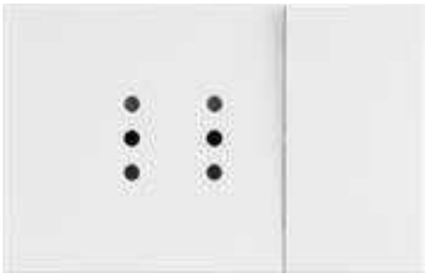
HK7327 10A / 120-250V 10A / 250V HK7327.3W 10A / 120-250V 10A / 250V
