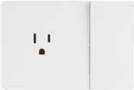
HS7213 10A / 120-250V 15A / 125V HS7213.3W 10A / 120-250V 15A / 125V
