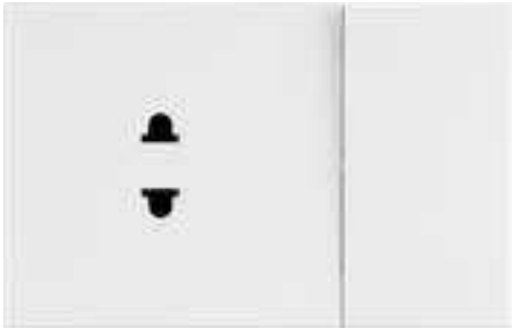
HK7212 10A / 120-250V 15A / 120-250V HK7212.3W 10A / 120-250V 15A / 120-250V
