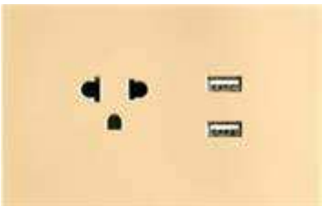
HK2296.MCHP 15A / 120-250V 2.1A / 5V TOMA USB-A
